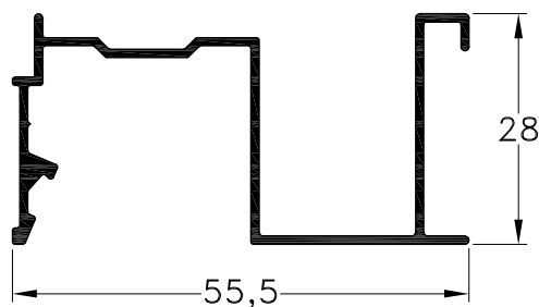
1010082 - Guía de Cortina Común Peso: 0,42 Kg/m. Largo Std.: 6.200 mm.
