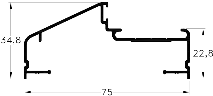
1010398 - Revestimiento Tubular Peso: 0,91 Kg/m. Largo Std.: 6.030 mm.
