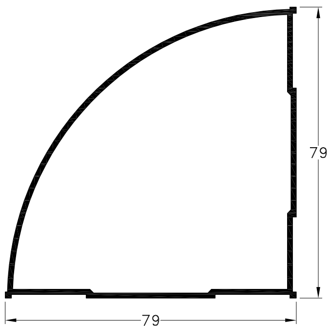
1010986 - Columna Curva a 90° Peso: 1,06 Kg/m. Largo Std.: 6.030 mm.
