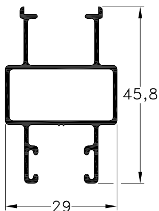
1010103 - Parante Lateral Peso: 0,46 Kg/m. Largo Std.: 6.030 mm.
