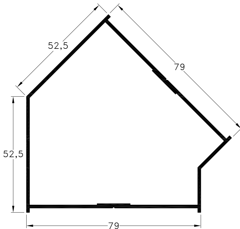
1010043 - Columna Acople a 45°
