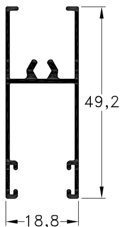
1010902 - Zócalo y Cabezal Peso: 0,38 Kg/m. Largo Std.: 6.030 mm.
