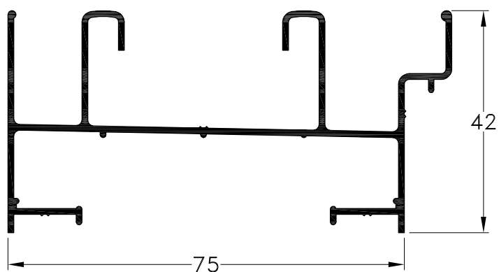
1010921 - Marco Peso: 1,00 Kg/m. Largo Std.: 6.030 mm.
