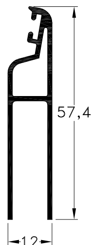
1010981 - Terminal Largo Peso: 0,45 Kg/m. Largo Std.: 6.030 mm.
