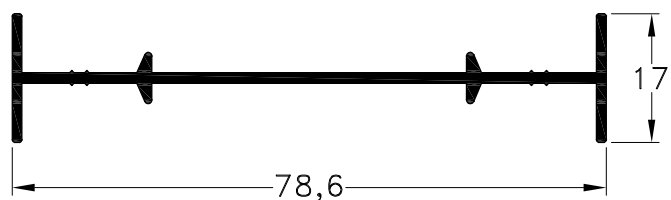
1010453 - Acople Recto Peso: 0,45 Kg/m. Largo Std.: 6.030 mm.
