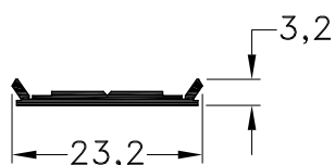
1010905 - Base Molduras Peso: 0,10 Kg/m. Largo Std.: 6.030 mm.
