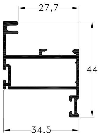
1010919 - Hoja Banderola Peso: 0,53 Kg/m. Largo Std.: 6.030 mm.
