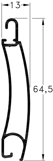
1010625 - Tablilla Cortina Común Peso: 0,42 Kg/m. Largo Std.: 6.200 mm. (Largo Opc.: 5.400 mm.)
