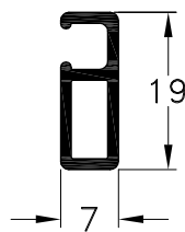
1010061 - Mosquitero Fijo Peso: 0,17 Kg/m. Largo Std.: 6.030 mm.
