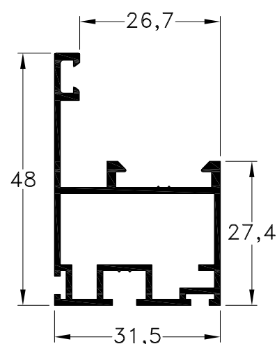
1040507 - Hoja Peso: 0,56 Kg/m. Largo Std.: 6.030 mm.
