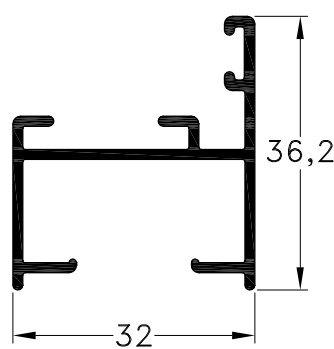
1010077 - Marco Simple Peso: 0,43 Kg/m. Largo Std.: 6.200 mm.
