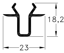
1040027 - Encuentro de Cuatro Hojas Peso: 0,18 Kg/m. Largo Std.: 6.030 mm.
