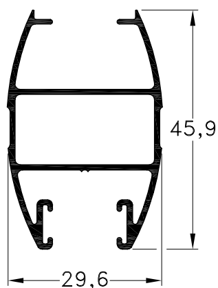
1010014 - Parante Lateral Moderno Peso: 0,51 Kg/m. Largo Std.: 6.030 mm.
