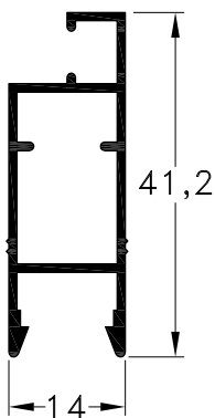
1010105 - Mosquitero Peso: 0,32 Kg/m. Largo Std.: 6.030 mm.
