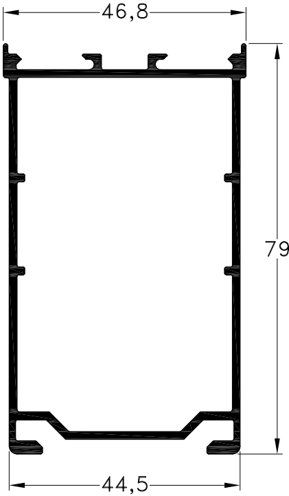
1010433 - Parante Peso: 1,13 Kg/m. Largo Std.: 6.200 mm. Largo Opc.: 4.500 mm.
