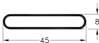
1010976 - Tablilla Fija Peso: 0,26 Kg/m. Largo Std.: 6.030 mm.
