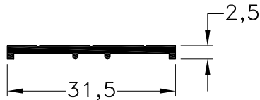
1010410 - Tapajunta Peso: 0,13 Kg/m. Largo Std.: 6.030 mm.
