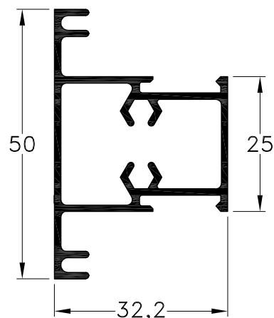
1010674 - Travesaño Peso: 0,63 Kg/m. Largo Std.: 6.030 mm.
