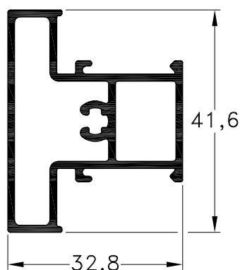
1011946 - Travesaño Angosto Peso: 0,67 Kg/m. Largo Std.: 6.030 mm.
