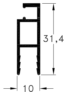
1010060 - Mosquitero Peso: 0,25 Kg/m. Largo Std.: 6.030 mm.
