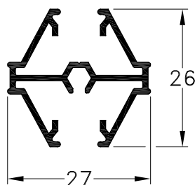
1010471 - Travesaño Peso: 0,32 Kg/m. Largo Std.: 6.030 mm.
