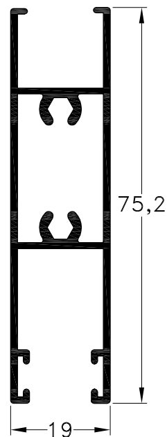
1010005 - Zócalo Alto Puerta Corrediza Peso: 0,81 Kg/m. Largo Std.: 6.030 mm.
