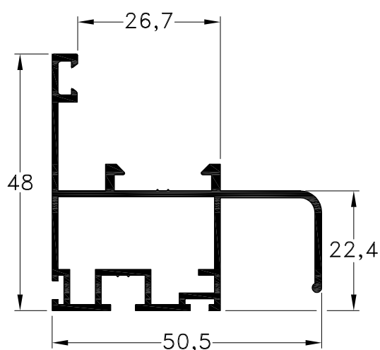
1040506 - Zócalo/Cabecal Peso: 0,69 Kg/m. Largo Std.: 6.030 mm.
