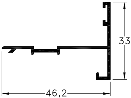
1010016 - Batiente Peso: 0,31 Kg/m. Largo Std.: 6.200 mm.
