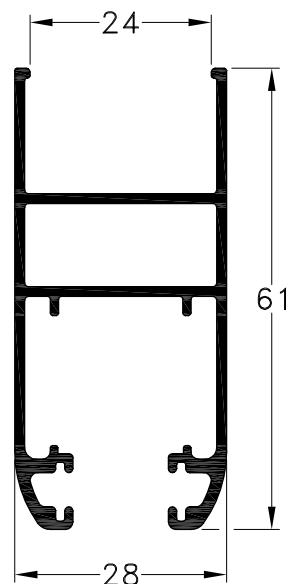
1040482 - Hoja D.V.H. Peso: 0,76 Kg/m. Largo Std.: 6.030 mm.
