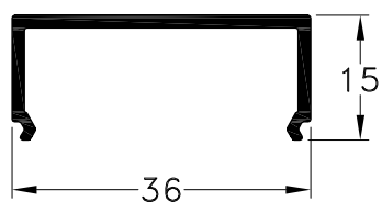
1010975 - Asiento Tablilla Fija 1010976 Peso: 0,26 Kg/m. Largo Std.: 6.030 mm.
