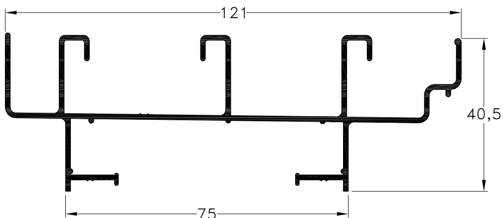
1010961 - Marco de Tres Guías Peso: 1,16 Kg/m. Largo Std.: 6.030 mm.
