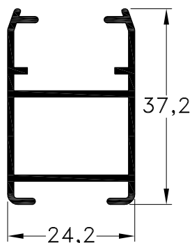
1010462 - Parante Peso: 0,45 Kg/m. Largo Std.: 6.030 mm.
