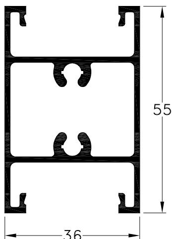
1010979 - Travesaño Peso: 0,99 Kg/m. Largo Std.: 6.030 mm.
