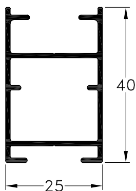
1010968 - Parante Peso: 0,48 Kg/m. Largo Std.: 6.030 mm.
