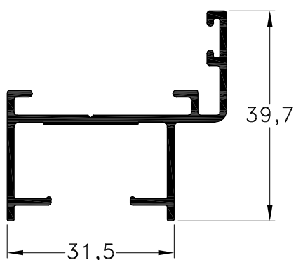
1010956 - Marco Angosto Peso: 0,50 Kg/m. Largo Std.: 6.200 mm.
