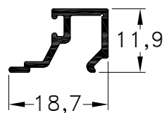
1010947 - Contravidrio Peso: 0,14 Kg/m. Largo Std.: 6.030 mm.
