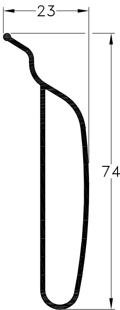
1010628 - Tablilla Cortina Regulable Peso: 0,48 Kg/m. Largo Std.: 6.030 mm. Largo Opc.: 5.400 mm.
