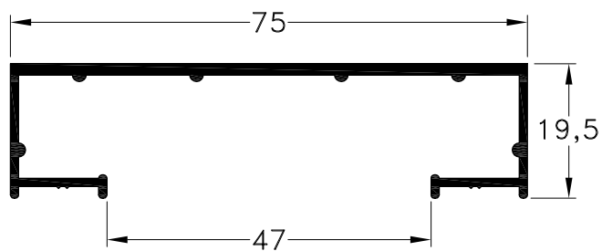
1010924 - Marco Recto Peso: 0,56 Kg/m. Largo Std.: 6.030 mm.
