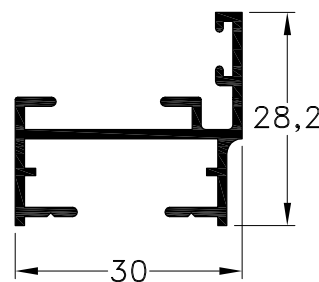
1010291 - Marco Raja Peso: 0,35 Kg/m. Largo Std.: 6.030
