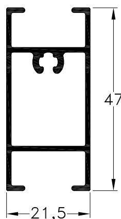
1010958 - Travesaño para Perfiles 1010968 y 1010969 Peso: 0,53 Kg/m. Largo Std.: 6.030 mm.
