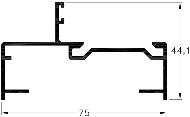
1010432 - Marco Peso: 0,79 Kg/m. Largo Std.: 6.200 mm.
