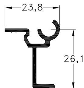
1040750 - Soporte Tapacinta Peso: 0,28 Kg/m. Largo Std.: 6.150 mm.
