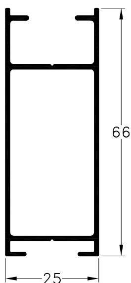
1010969 - Parante Peso: 0,63 Kg/m. Largo Std.: 6.200 mm.
