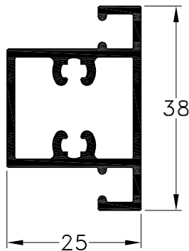
1010089 - Travesaño Puerta Mosquitero de Rebatir Peso: 0,61 Kg/m. Largo Std.: 6.030 mm.
