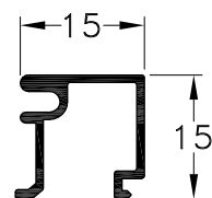
1010908 - Contravidrio V.S. Peso: 0,16 Kg/m. Largo Std.: 6.030 mm.
