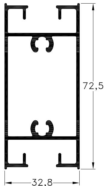
1011945 - Travesaño Peso: 1,07 Kg/m. Largo Std.: 6.030 mm.
