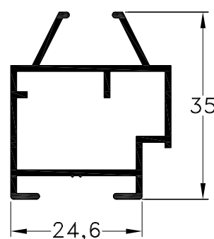
1010290 - Hoja Raja Peso: 0,44 Kg/m. Largo Std.: 6.030
