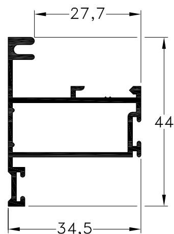
1010918 - Hoja Ventiluz Peso: 0,51 Kg/m. Largo Std.: 6.030 mm.
