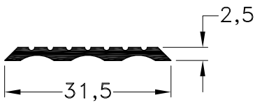
1010066 - Tapacanto Peso: 0,15 Kg/m. Largo Std.: 6.030 mm.
