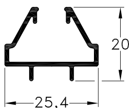
1010092 - Perimetral Peso: 0,23 Kg/m. Largo Std.: 6.030 mm.
