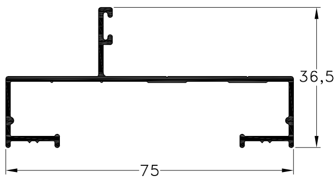
1010427 - Marco Puerta de Rebatir 45 mm. Peso: 0,58 Kg/m. Largo Std.: 6.200 mm.
