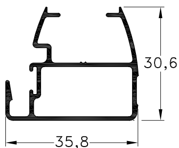
1010015 - Parante Central Moderno Peso: 0,41 Kg/m. Largo Std.: 6.030 mm.
