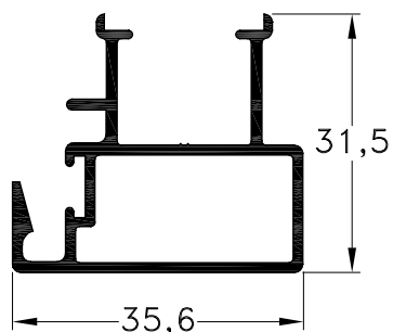
1010084 - Parante Central Peso: 0,50 Kg/m. Largo Std.: 6.030 mm.
