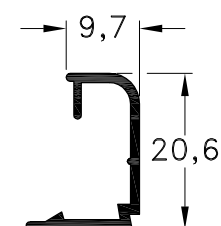
1040510 - Contravidrio D.V.H. Peso: 0,15 Kg/m. Largo Std.: 6.030 mm.
