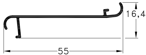
1010926 - Tablilla Fija Peso: 0,21 Kg/m. Largo Std.: 6.030 mm.
