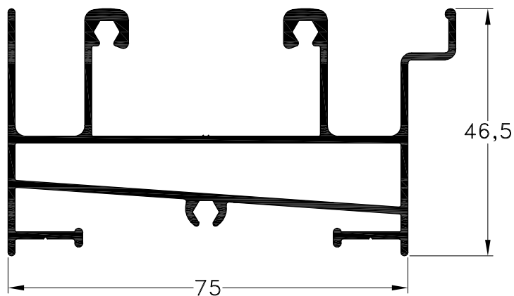
1010920 - Umbral con Caja de Agua Peso: 1,35 Kg/m. Largo Std.: 6.030 mm.
