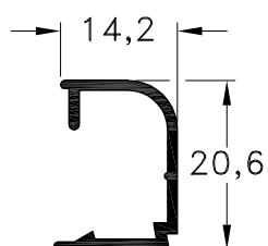
1040508 - Contravidrio V.S. Peso: 0,17 Kg/m. Largo Std.: 6.030 mm.
