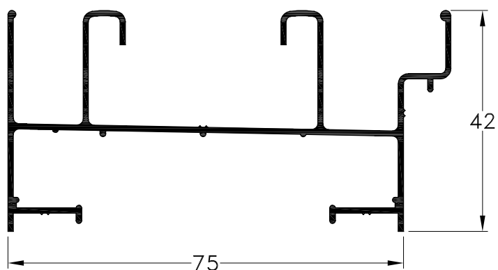
1010901 - Marco Liviano Peso: 0,75 Kg/m. Largo Std.: 6.030 mm.
