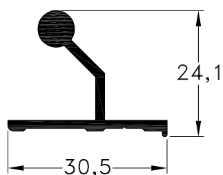
1010915 - Bisagra Peso: 0,33 Kg/m. Largo Std.: 6.030 mm.
