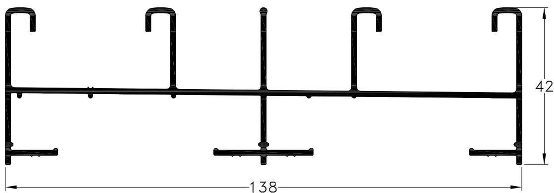
1010960 - Marco de Cuatro Guías Peso: 1,53 Kg/m. L. Std.: 6.030 mm.
