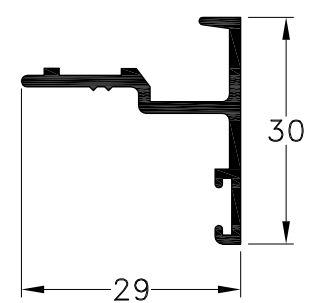
1010093 - Batiente Peso: 0,28 Kg/m. Largo Std.: 6.200 mm.
