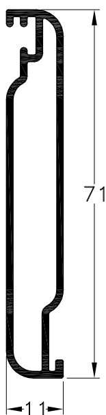
1010096 - Tablilla Peso: 0,59 Kg/m. Largo Std.: 6.030 mm.
