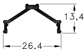
1010903 - Moldura Puerta Placa Peso: 0,16 Kg/m. Largo Std.: 6.030 mm.
