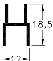
1010582 - Calce Tapaluz Peso: 0,15 Kg/m. Largo Std.: 6.020 mm.
