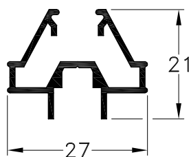
1010470 - Perimetral Peso: 0,27 Kg/m. Largo Std.: 6.030 mm.
