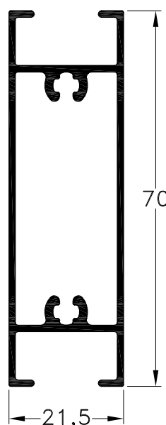
1010959 - Travesaño Alto para Perfiles 1010968 y 1010969 Peso: 0,74 Kg/m. Largo Std.: 6.030 mm.
