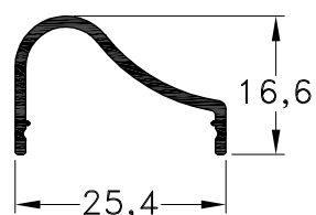
1010904 - Moldura Puerta Placa Peso: 0,16 Kg/m. Largo Std.: 6.030 mm.
