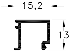
1010034 - Contravidrio Peso: 0,14 Kg/m. Largo Std.: 6.030 mm.
