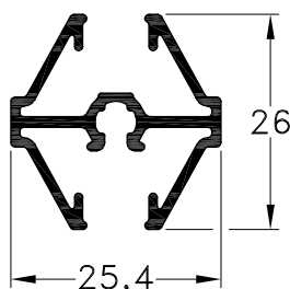
1010091 - Travesaño Peso: 0,35 Kg/m. Largo Std.: 6.030 mm.
