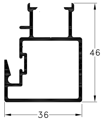
1010954 - Parante Central Peso: 0,68 Kg/m. Largo Std.: 6.200 mm.
