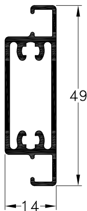
1010106 - Travesaño Peso: 0,49 Kg/m. Largo Std.: 6.030 mm.
