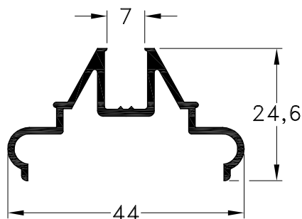
1011964 - Aplique Perimetral 7 mm. Peso: 0,35 Kg/m. Largo Std.: 6.030 mm.
