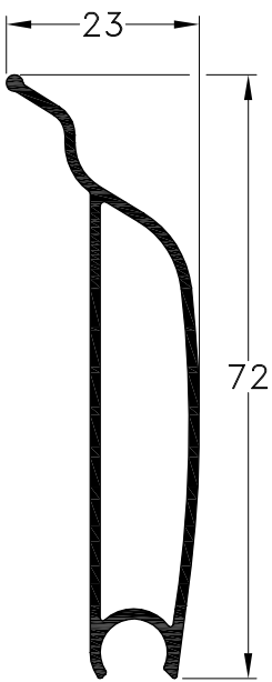
1010627 - Primera Tablilla Cortina Regulable Peso: 0,49 Kg/m. Largo Std.: 6.030 mm.
