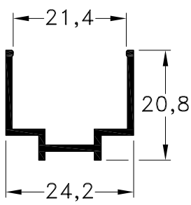
1010553 - Adaptador D.V.H. Peso: 0,21 Kg/m. Largo Std.: 6.030 mm.
