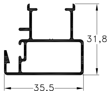
1010104 - Parante Central Peso: 0,42 Kg/m. Largo Std.: 6.030 mm.
