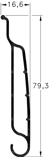
1010983 - Primera Tablilla Cortina Regulable Rosario Peso: 0,53 Kg/m. Largo Std.: 6.200 mm.
