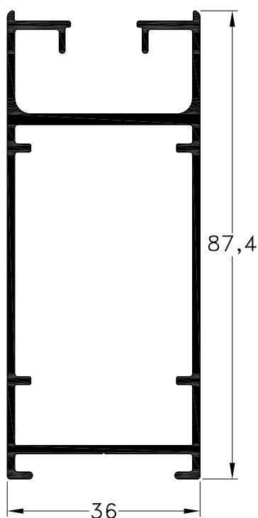
1011943 - Parante Ancho Peso: 1,16 Kg/m. Largo Std.: 6.200 mm. Largo Opc.: 4.500 mm.
