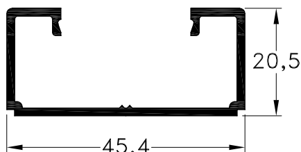
1010583 - Adaptador Puerta de Rebatir 45 mm. Peso: 0,44 Kg/m. Largo Std.: 6.020 mm.
