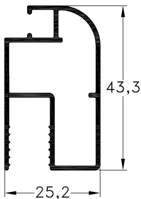
1060108 - Mosquitero Peso: 0,47 Kg/m. Largo Std.: 6.030 mm.
