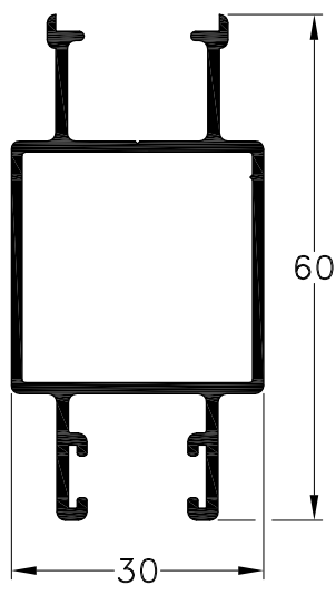
1010953 - Parante Lateral Peso: 0,70 Kg/m. Largo Std.: 6.200 mm.
