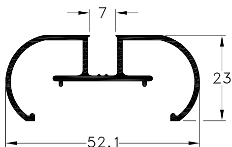
1010940 - Aplique Perimetral 7 mm. Peso: 0,48 Kg/m. Largo Std.: 6.030 mm.
