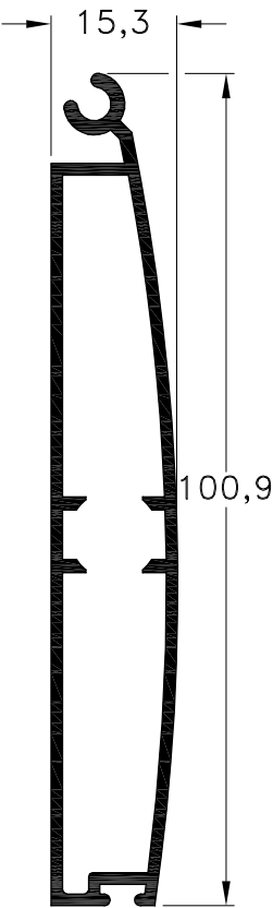
1010626 - Zócalo Cortina Regulable Peso: 0,90 Kg/m. Largo Std.: 6.030 mm.
