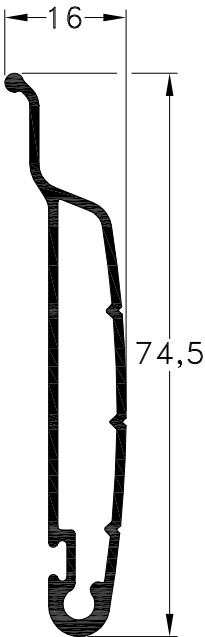
1010899 - Tablilla Cortina Regulable Rosario Peso: 0,53 Kg/m. Largo Std.: 6.200 mm. (Largo Opc.: 5.400 mm.)
