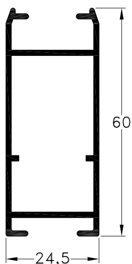
1010463 - Parante Peso: 0,56 Kg/m. Largo Std.: 6.200 mm.
