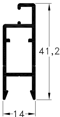
1010085 - Mosquitero Peso: 0,41 Kg/m. Largo Std.: 6.030 mm.
