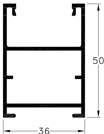
1010977 - Hoja Peso: 0,79 Kg/m. Largo Std.: 6.030 mm.
