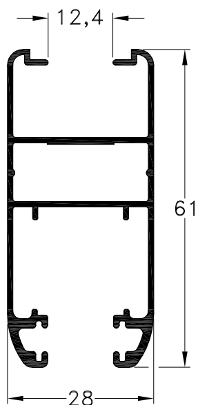
1040481 - Hoja V.S. Peso: 0,70 Kg/m. Largo Std.: 6.030 mm.
