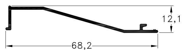
1010449 - Tablilla Fija Peso: 0,26 Kg/m. Largo Std.: 6.030 mm.
