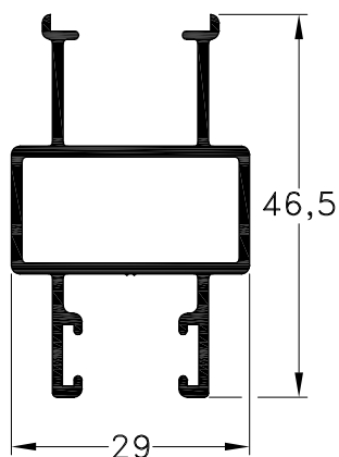
1010083 - Parante Lateral Peso: 0,56 Kg/m. Largo Std.: 6.030 mm.
