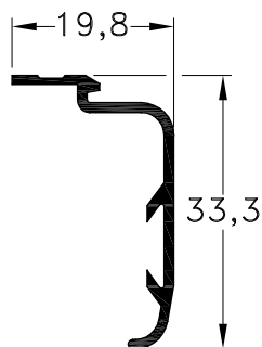
1010709 - Contramarco Peso: 0,19 Kg/m. Largo Std.: 6.150 mm.
