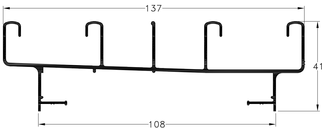
1010955 - Marco de Cuatro Guías Peso: 1,17 Kg/m. L. Std.: 6.030 mm.
