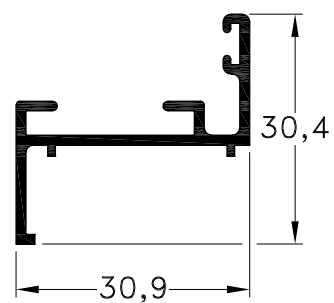
1010048 - Marco Hoja Secundaria Puerta de Rebatir 36 mm. Peso: 0,30 Kg/m. Largo Std.: 6.020 mm.
