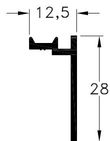
1010441 - Contramarco Peso: 0,18 Kg/m. Largo Std.: 6.150 mm.
