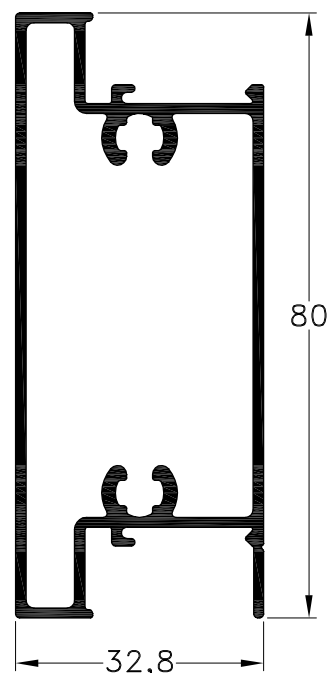
1011947 - Zócalo-Travesaño Peso: 1,07 Kg/m. Largo Std.: 6.030 mm.
