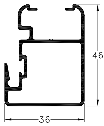
1010019 - Parante Central Reforzado Moderno Peso: 0,73 Kg/m. Largo Std.: 6.200 mm.
