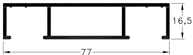
1010715 - Premarco Peso: 0,70 Kg/m. Largo Std.: 6.150 mm.
