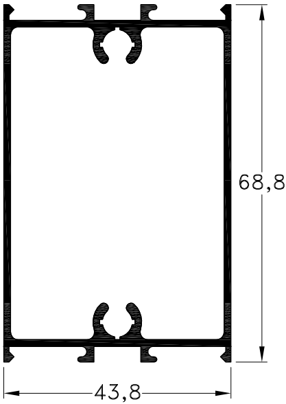
1010429 - Travesaño Peso: 1,01 Kg/m. Largo Std.: 6.030
