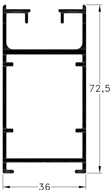
1011944 - Parante Angosto Peso: 1,05 Kg/m. Largo Std.: 6.200 mm. Largo Opc.: 4.500 mm.
