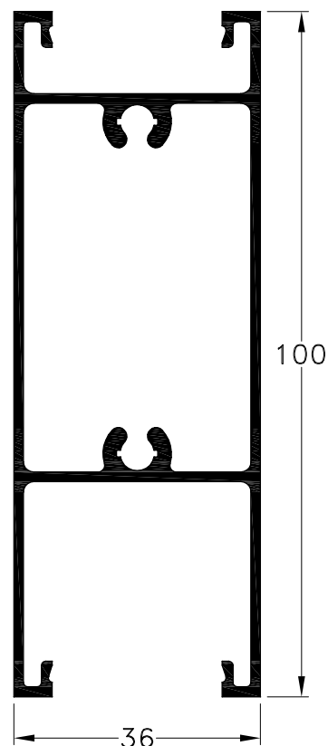
1010978 - Travesaño Reforzado Peso: 1,33 Kg/m. Largo Std.: 6.030 mm.
