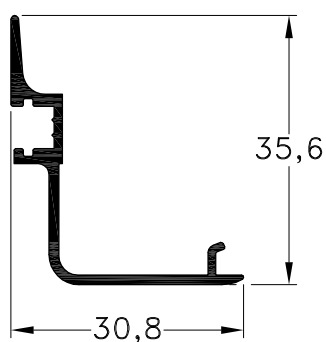
1040026 - Encuentro de Hojas Peso: 0,27 Kg/m. Largo Std.: 6.030 mm.
