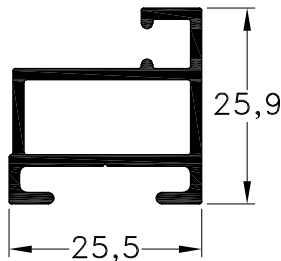
1010090 - Hoja Puerta Mosquitero de Rebatir Peso: 0,43 Kg/m. Largo Std.: 6.030 mm.
