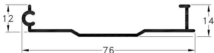
1010122 - Tapacinta Móvil Peso: 0,29 Kg/m. Largo Std.: 6.030 mm.
