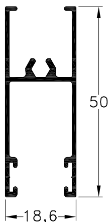
1010922 - Zócalo y Cabezal Peso: 0,52 Kg/m. Largo Std.: 6.030 mm.
