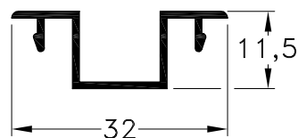
1010581 - Adaptador Terminal Peso: 0,17 Kg/m. Largo Std.: 6.020 mm.
