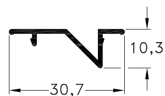
1040509 - Tapa Peso: 0,14 Kg/m. Largo Std.: 6.030 mm.
