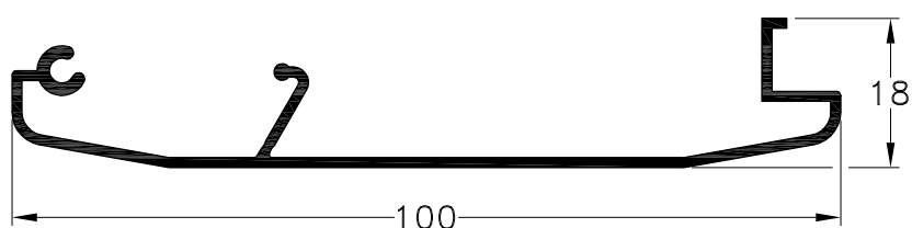
1050716 - Tapacinta Peso: 0,52 Kg/m. Largo Std.: 6.150 mm.
