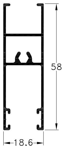
1010023 - Zócalo y Cabezal Peso: 0,50 Kg/m. Largo Std.: 6.030 mm.
