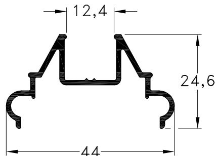
1011948 - Aplique Perimetral 12 mm. Peso: 0,35 Kg/m. Largo Std.: 6.030 mm.
