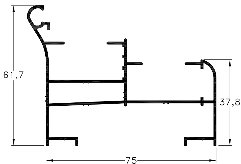
1040505 - Marco Peso: 0,97 Kg/m. Largo Std.: 6.030 mm.
