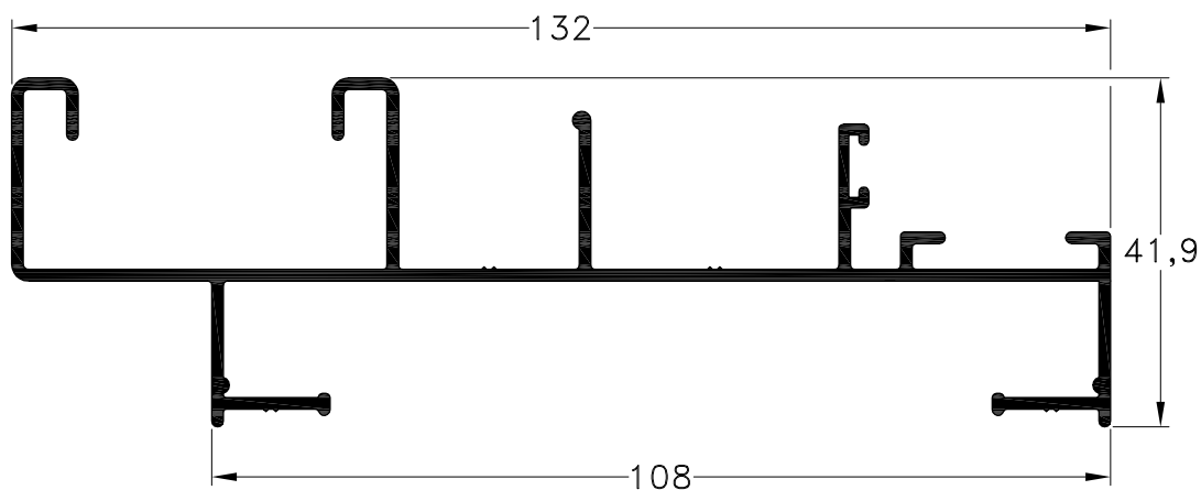
1010088 - Marco Unificado con Postigón Rebatible Peso: 1,21 Kg/m. L. Std.: 6.030 mm.
